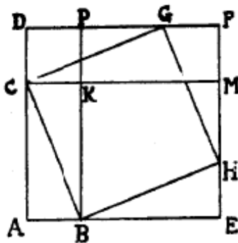
Supponiamo che nel triangolo rettangolo ABC (fig. 15) sia l'angolo retto ed AC il cateto maggiore. Sul prolungamento del cateto AC prendiamo CD = AB e sul prolungamento di AB prendiamo BE = AC . Ne segue AE = AD . Per C e per D conduciamo dalla parte di B rispetto ad AD le semirette perpendicolari alla AD e prendiamo su esse DP = CK = AB ; e congiungiamo K con P e con B.
