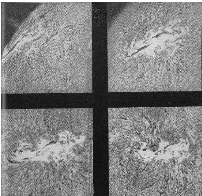
TAV. VII. – Evoluzione d'una macchia solare. (Spettografia ottenuta all'osservatorio del Monte Wilson).
