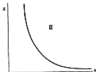
Fig. 9. \lambda < 0 , \mu < 0
