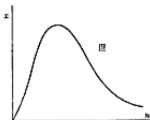
Fig. 10. \lambda > 0 , \mu < 0
