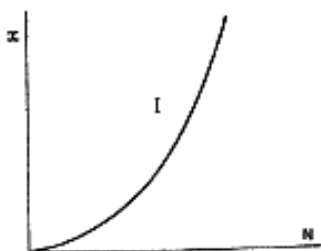
Fig. 8. \lambda > 0 , \mu > 0
