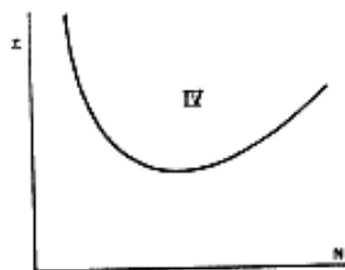
Fig. 11. \lambda < 0 , \mu > 0
