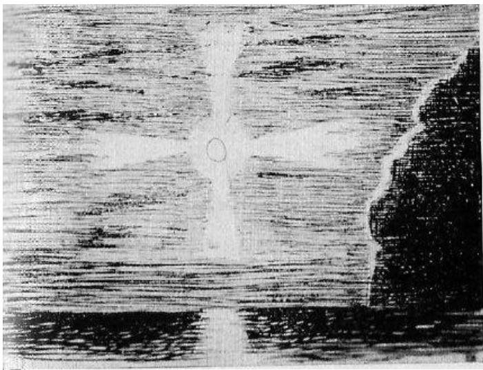
TAV. IX – Anormale rifrazione osservata nel Golfo di Aden dalla nave Clydebank il 10 maggio 1934 al tramonto. – Sotto: Alone osservato sull'Oceano Atlantico Nord dalla nave Orduna il 12 luglio 1935.
