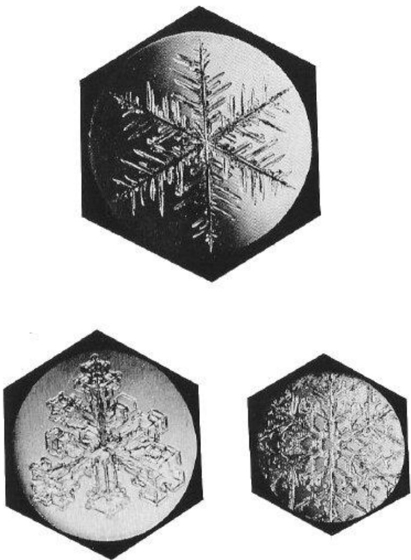
TAV. XIX – Microfotografie di cristalli di neve.
