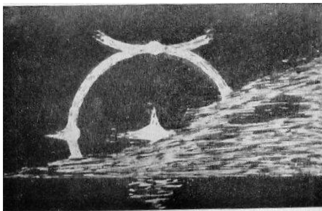
TAV. VIII – Sopra: Alone lunare osservato sul Mediterraneo dalla nave Cerintbus il 7 nov. 1932. – Sotto: Alone lunare osservato sull'Oceano Atlantico Nord dalla nave Montcalm il 26 febbraio 1934.
