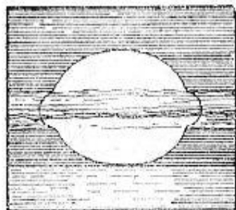
Deformazioni delle immagini della Luna al sorgere.
