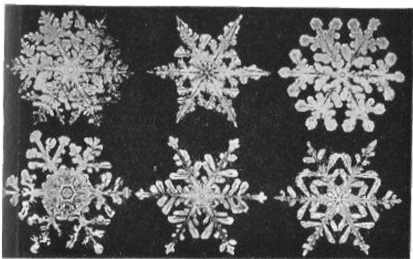
TAV. XVII – I cristalli di neve disegnati da W. A. Bentley. Forme a
