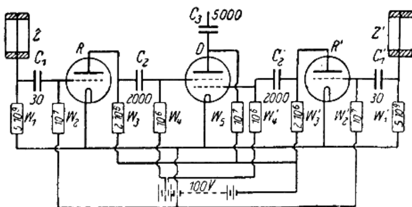
Fig. 77. – Disposizione per funzionamento in coincidenza di due contatori di GEIGER e MÜLLER (Z e Z').
