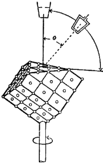
Fig. 21. – Schema della disposizione per lo studio della diffrazione elettronica. Il cristallo di nickel ha al di sopra il cannonecino per lancio degli elettroni e da un lato il pozzetto di FARADAY che riceve gli elettroni diffratti dal cristallo.
