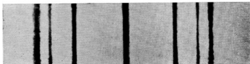
b) Spettro di velocità per elettroni ottenuti da argento eccitato con la riga K del tungsteno (M. DE BROGLIE).
