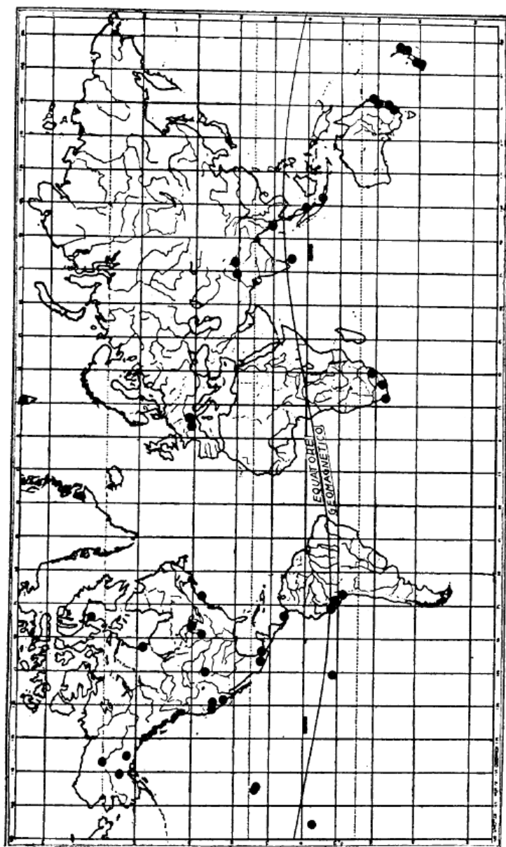
Fig. 79. – Cartina con le stazioni (punti segnati ●) sede di osservatori per lo
