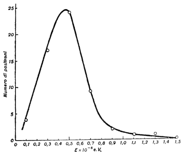
Fig. 82. — La distribu- zione delle energie dei positroni emessi da radio-fosfo- ro.
