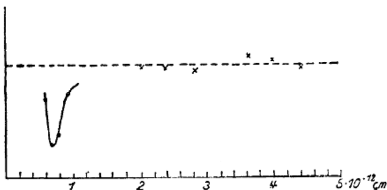
Fig. 63. – Diffusione di particelle \alpha in lastrine di Mg (punti e curva) e Ag (crocette e punteggiata) sotto l'angolo di 135^\circ . Sull'asse delle ordinate sono i rapporti fra il numero delle particelle diffuse secondo l'esperienza e quello calcolato in base alla legge di Coulomb. Sull'asse delle ascisse sono le distanze minime dal nucleo a cui le particelle sono arrivate. Si vede che le particelle diffuse da Ag che si avvicinano meno al nucleo diffondono come vuole la teoria. Quelle che hanno traversato Mg a distanze inferiori a 10^{-12} cm presentano diffusione anormale.
