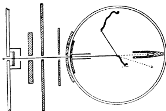
Fig. 17. – Schema delle fotografie ottenute alla camera del WILSON per l'effetto Compton. La
