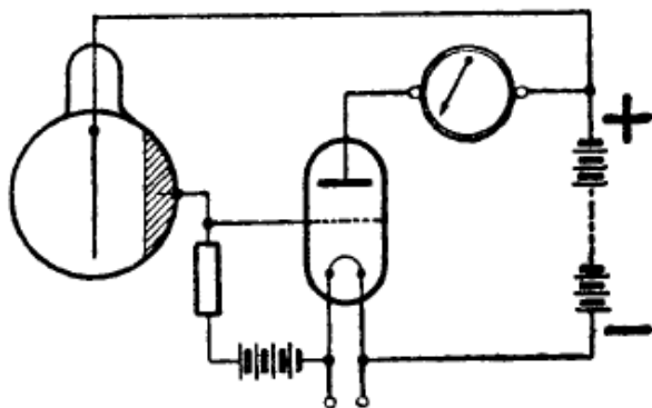
Fig. 14. – Schema di circuito pel funzionamento di una cella fotoelettrica.
