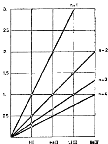
Fig. 48. – Schema del MOSELEY pei livelli energetici esterni degli atomi che hanno un solo elettrone (idrogeno, elio, ionizzato una volta, litio doppiamente ionizzato, berillio ionizzato tre volte).
