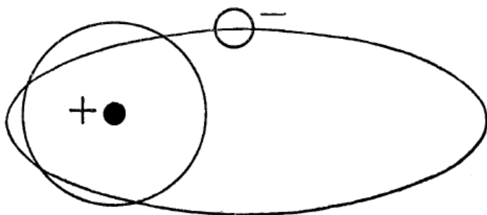
Fig. 40. – L'atomo di RUTHERFORD e BOHR.
