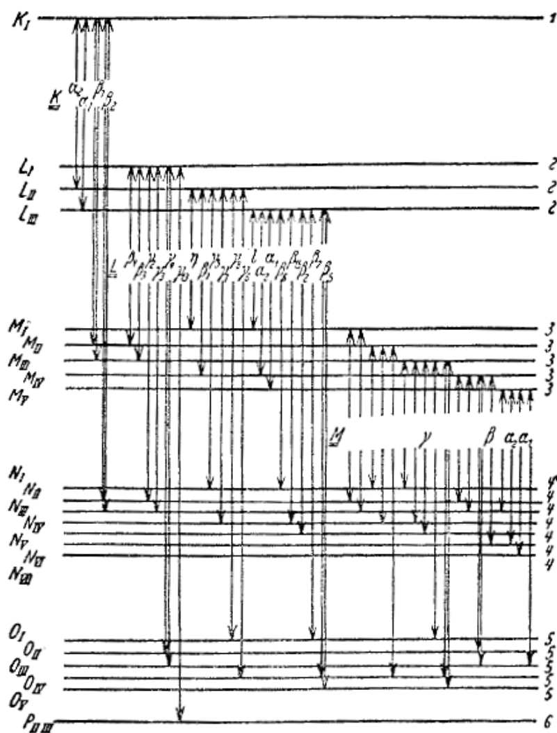
Fig. 46. – Schema dei livelli interni dell'uranio. In alto è il livello ( K ) più prossimo al nucleo. Le linee a doppia freccia rappresentano le transizioni possibili fra di essi e corrispondono quindi alle radia-
