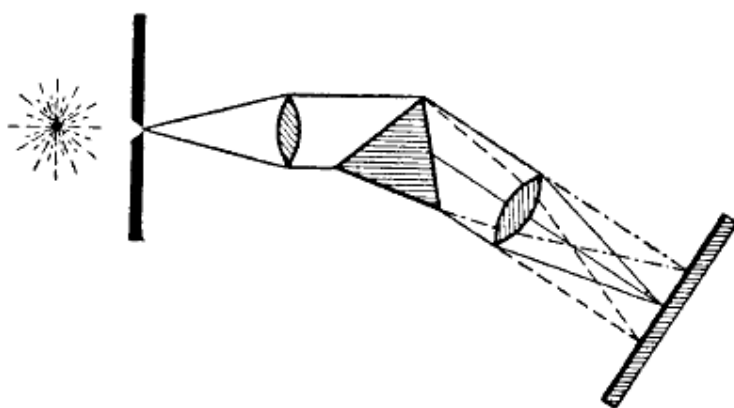
Fig. 1. – Schema del percorso dei raggi luminosi nello spettroscopio ottico. La sorgente illumina una fenditura, le cui immagini, diversamente colorate dopo il prisma, sono focheggiate su una lastra.
