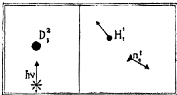
Fig. 74. – Schema illustrativo della scissione del diplogeno colpito da raggi \gamma .
