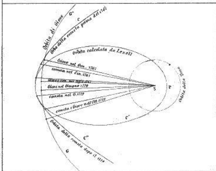
Orbite della Cometa del 1770
