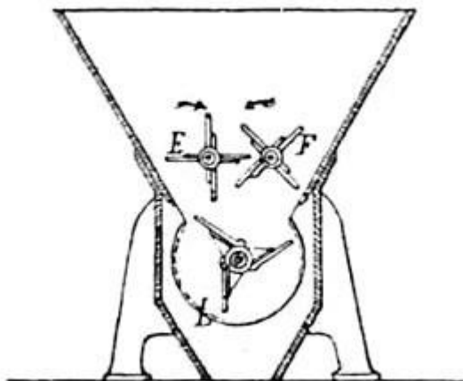
Sezione trasversale della diraspatrice Lindemann.
