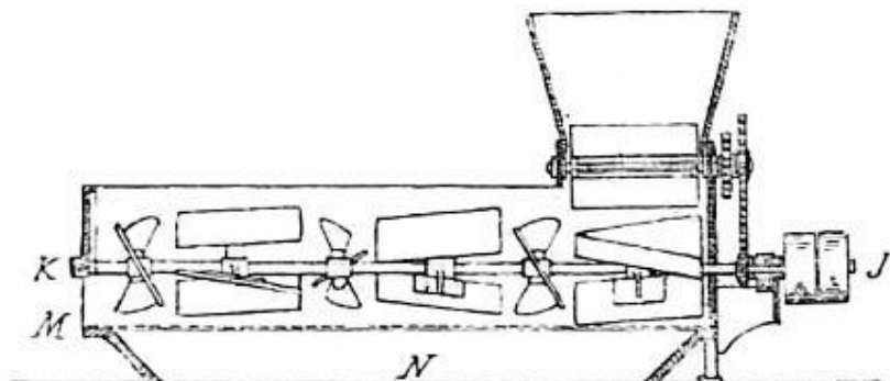
Sezione longitudinale della diraspatrice Lindemann a vapore.
