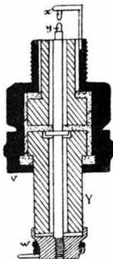
Fig. 20. Candela Bisson.
