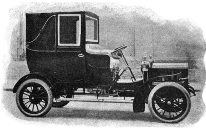
Fig. 106. — Vettura a vapore 18 HP White Landaulet.
