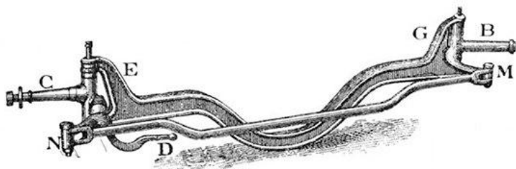
Fig. 73. Sterzo della vettura Rapid .
