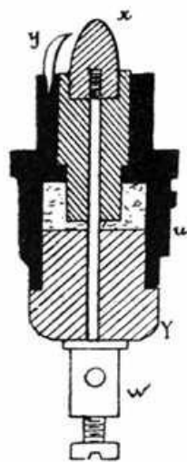
Fig. 19. Candela Reclus.
