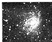
Fig. 2 H. 1, 1, 2 Cephei
