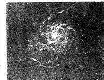
Fig. 9 M. 74 Piscium
