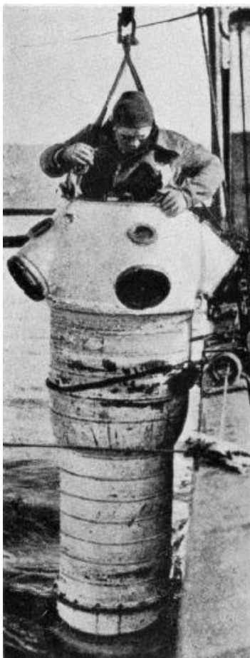
Sistema di scafandro rigido (Scafandro usato dalla Sorima di Genova)
