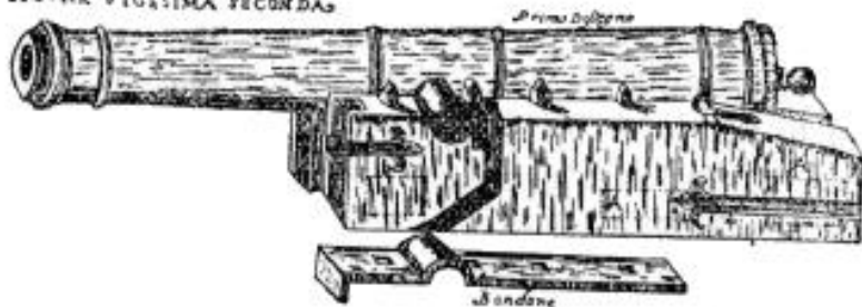
Tipo di cannone navale fisso alla nave.
