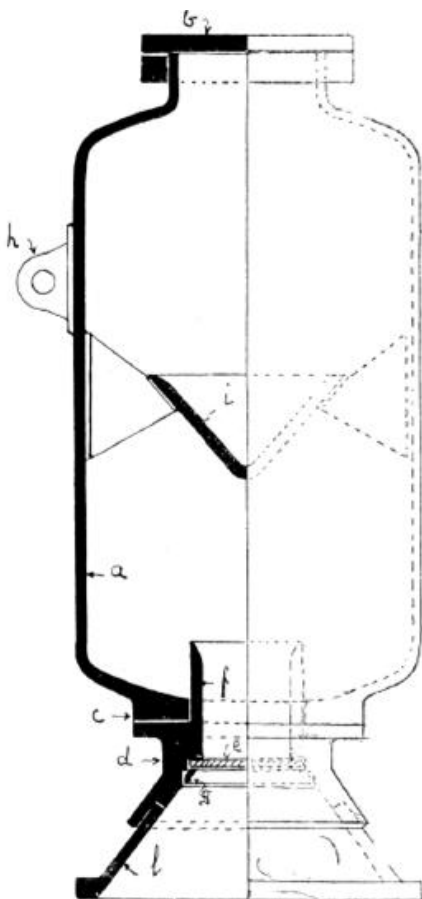
Sezione dello stesso (Ufficio Brevetti Barzanò e Zanardo). (Pag. 349)
